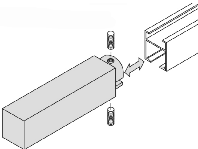
Befestigung Endstück
