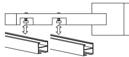
Montage Wandträger 2-läufig
