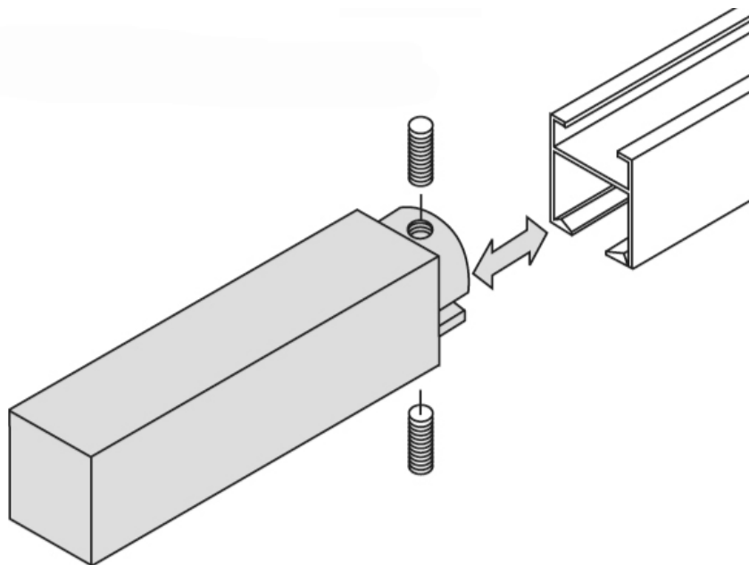
Befestigung Endstück
