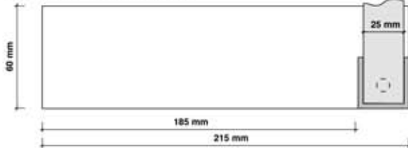
Standfuß Boden
