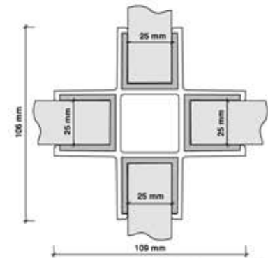
Kreuz-Verbinder
