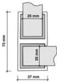
Eckverbinder
