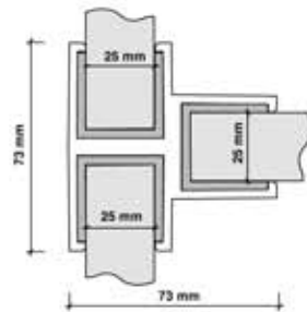
T-Verbinder
