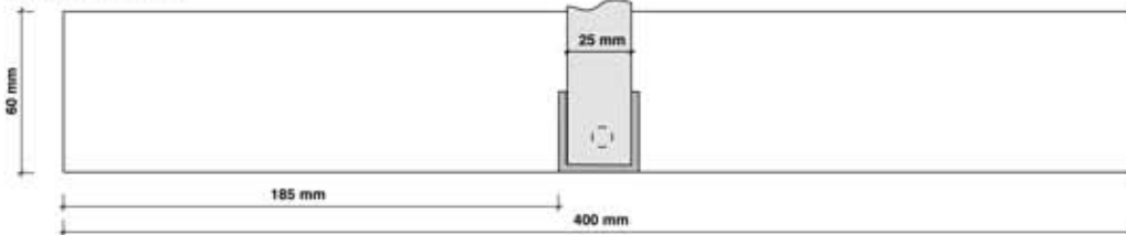
Eckverbinder
